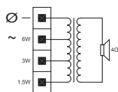
Schemat połączeń głośników LB1-UW06x-x
