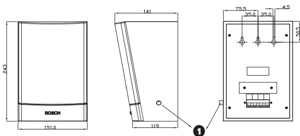
Wymiary głośników LB1-UW06x-x z regulacją głośności (1)
