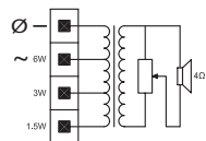
Schemat połączeń głośników LB1-UW06V-x
