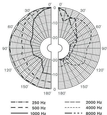
Charakterystyka kierunkowości w płaszczyźnie pionowej (pomiar szumem różowym)
