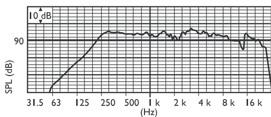
Pasmo przenoszenia
