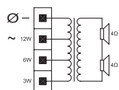
Schemat połączeń
