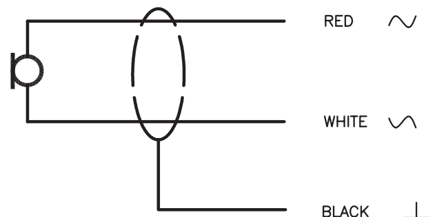
Schemat połączeń
